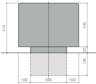
VISTA FRENTE
