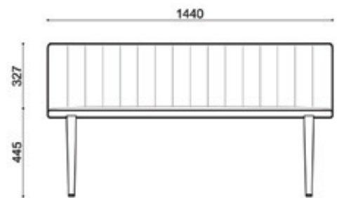
VISTA FRENTE
